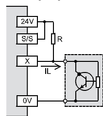
Circuito a logica negativa NPN (Sink)
