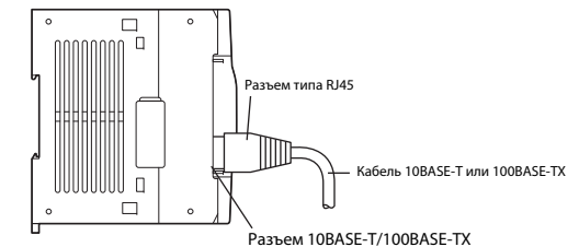
Разъем 10BASE-T/100BASE-TX
