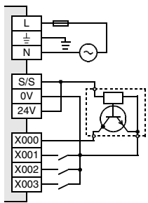
Minusschaltende Geber
