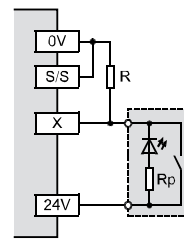
Plusschaltend (Source)
