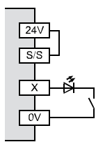
Circuito a logica negativa NPN (Sink)
