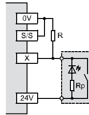
переключение на плюс (Source)
