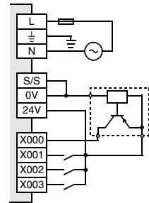
Датчик, переключающий на плюс (Source)
