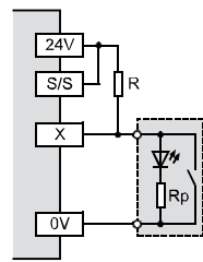
Minusschaltend (Sink)
