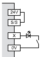
À commutation négative (Sink)
