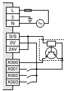
Trasduttore a logica negativa (NPN)
