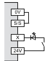
переключение на плюс (Source)
