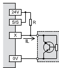
Minusschaltend (Sink)
