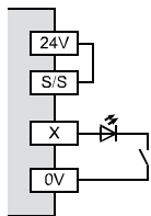
переключение на минус (Sink)
