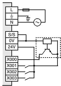
Plusschaltende Geber
